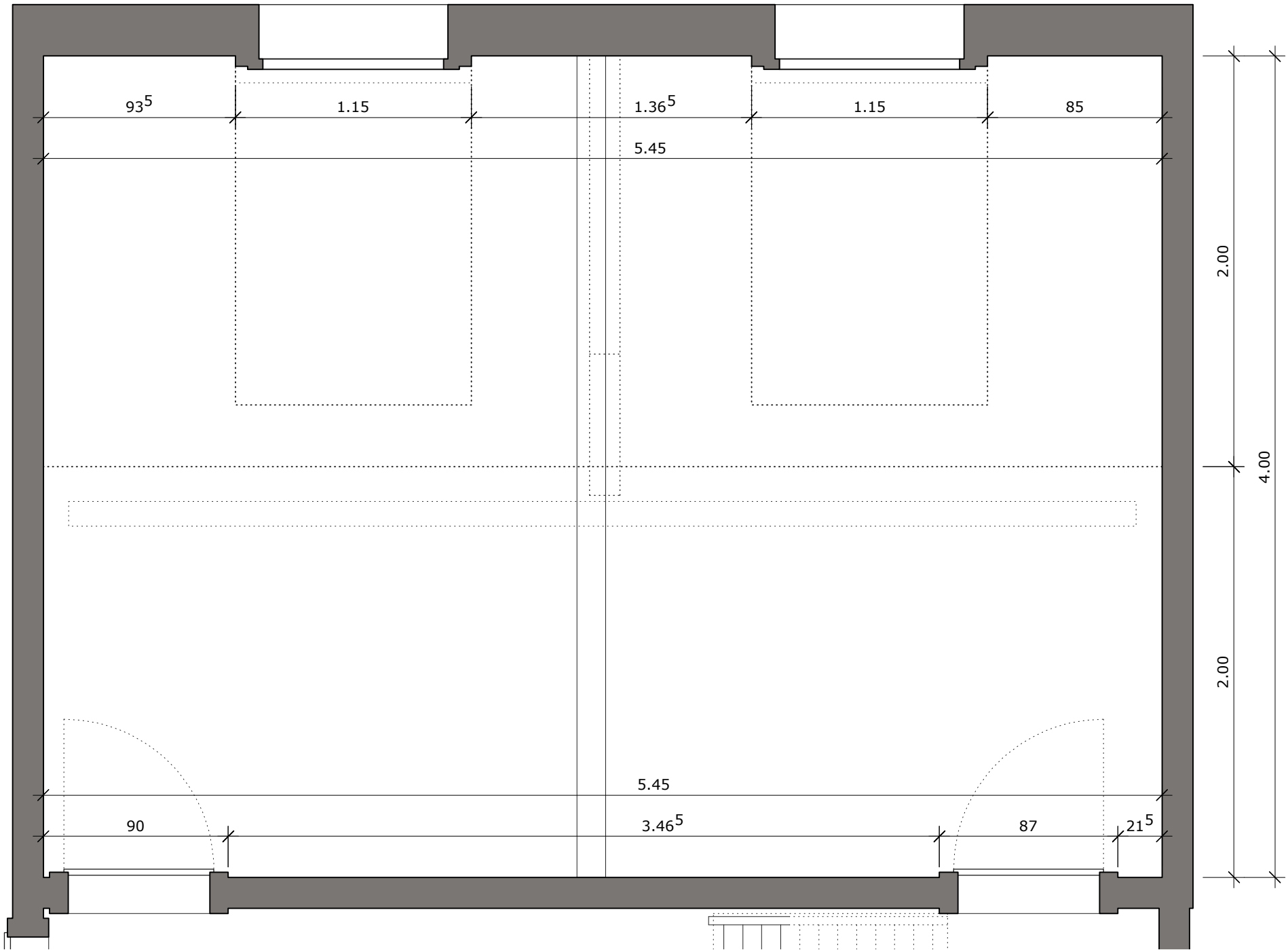
GRUNDRISS KUNSTZIMMER 1:25
